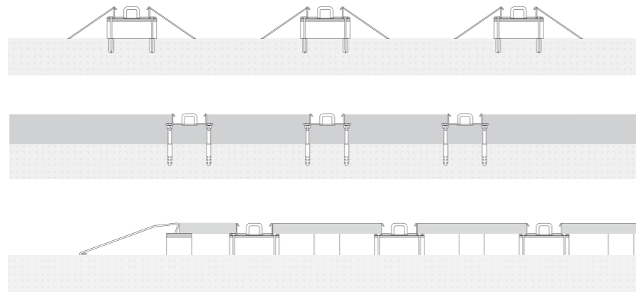
^ Rail implantation Implantación del sistema de raíles Système de rails
